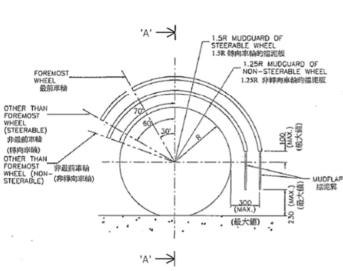
SECTION 'A' - 'A' 'A'-'A' 切面
