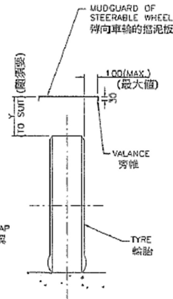
SECTION 'A' - 'A' 'A'-'A' 切面
