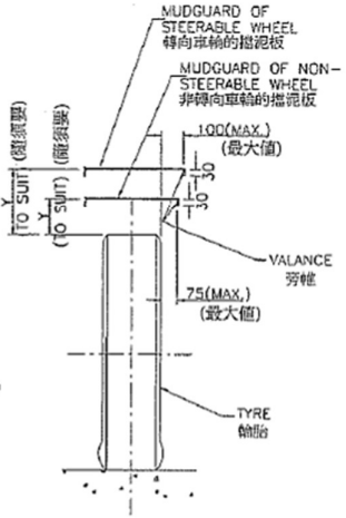
SECTION 'A' - 'A' 'A'-'A' 切面
